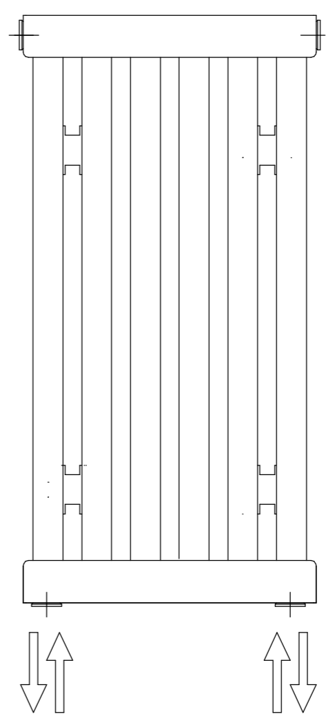
Размеры для подключения нижнее ЛП
