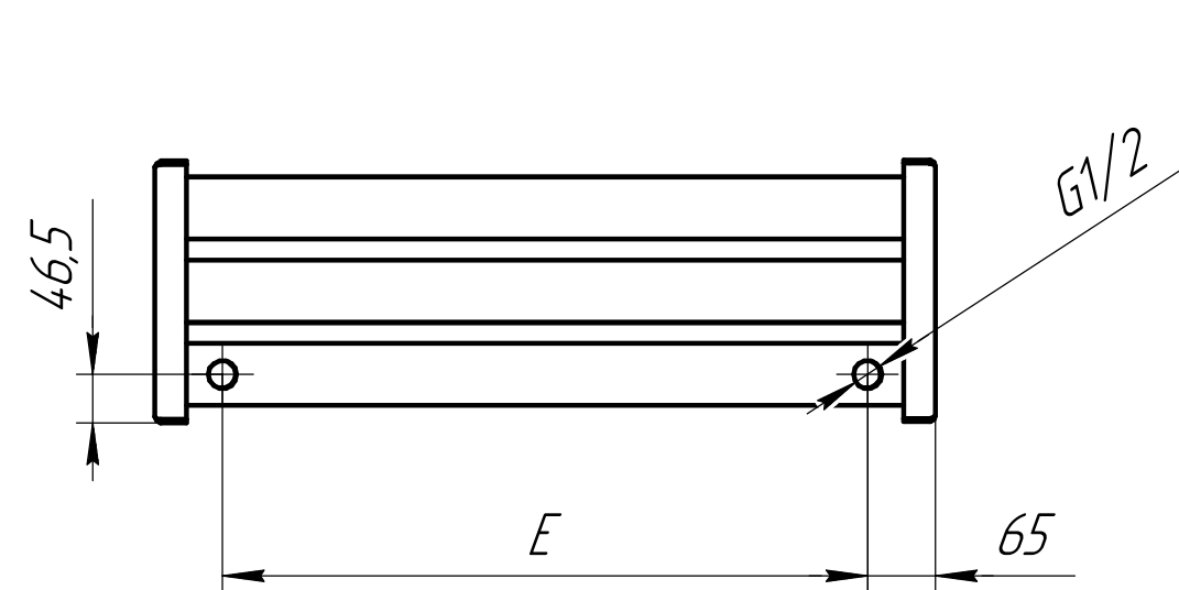
Размеры под подключение ЛП (вид снизу)
