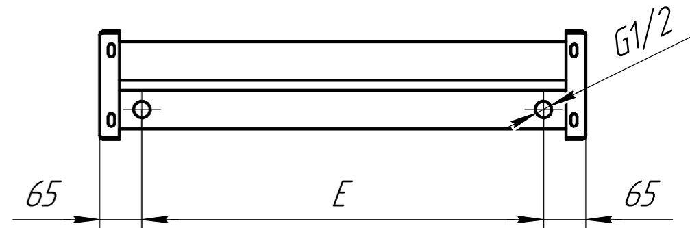
Размеры под подключение ЛП (вид снизу)
